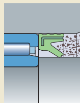
Hauptlippe nach außen gerichtet
