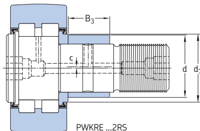
PWKRE ...2RS (PWKR ...2RS ohne Exzenterring)
