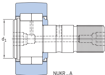
NUKR .. A (NUKRE ... A hat einen Exzenterring)
