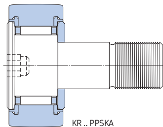
KR .. PPSKA
