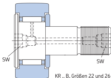
KR .. B, Größen 22 und 26 (KR .. PPA, Größen 22 und 26, mit Axialgleitscheiben)
