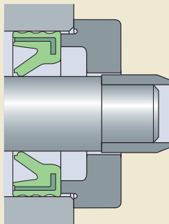
Einbauwerkzeug
