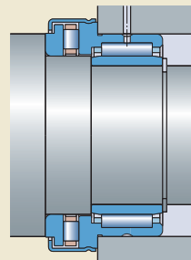
Nadel-Axial-Zylinderrollenlager, Reihe NKXR .. Z, kombiniert mit einem Innenring
