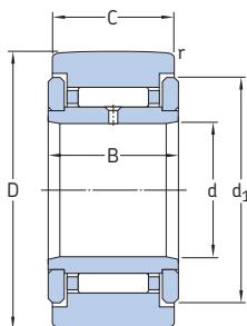
NATR.
