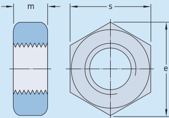
Sechskantmuttern
