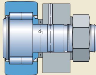
Abgestützter Bordring
