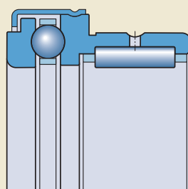
NKX .. Z
