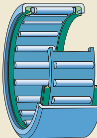
HK ...2RS
