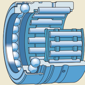
Reihe NX
