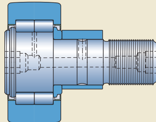
NUKRE .. A
