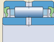
NA 49...2RS
