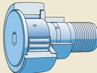
Kurvenrolle mit Exzenterring
