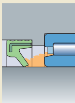
Hauptlippe nach innen gerichtet
