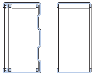
BK .. RS
