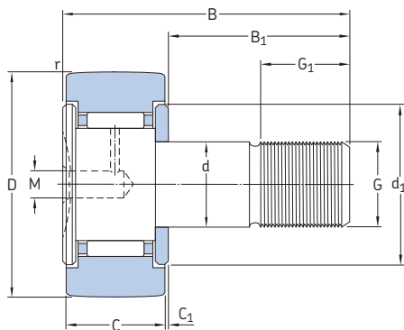
KR, Größen 16 und 19 (KR .. PPA, Größen 16 und 19, mit Axialgleitscheiben)
