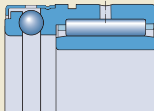
Reihe NX
