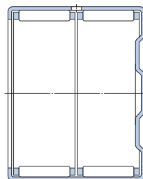
BK (zweireihig)
