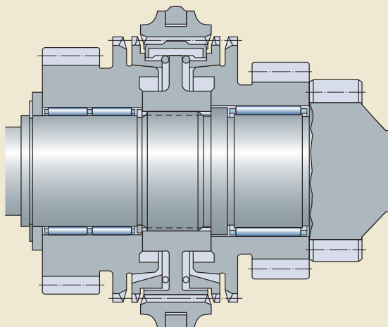
Lageranordnung mit geschlitzten Nadelkränzen
