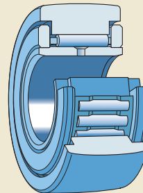
Stützrolle mit Bordscheiben
