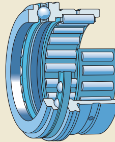
Reihe NKX
